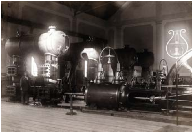
Dampfmaschinen im Pumpwerk Zell, heutiges Wasserwerk, um 1900
